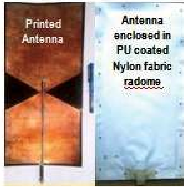
अनुरूपी ब्रॉडबैंड मुद्रित ऐंटेना
